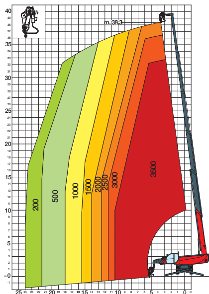
W 3,5 Winch 3,5 ton
