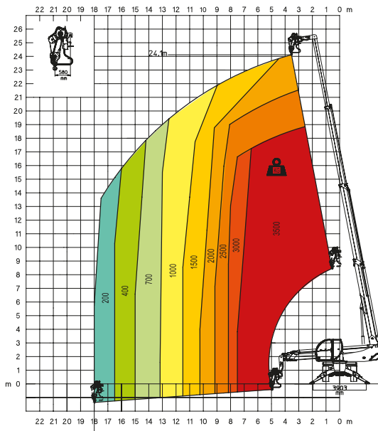
W 3,5 winch 3,5 ton
