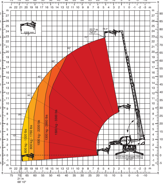
Jib winch 1.500 kg
